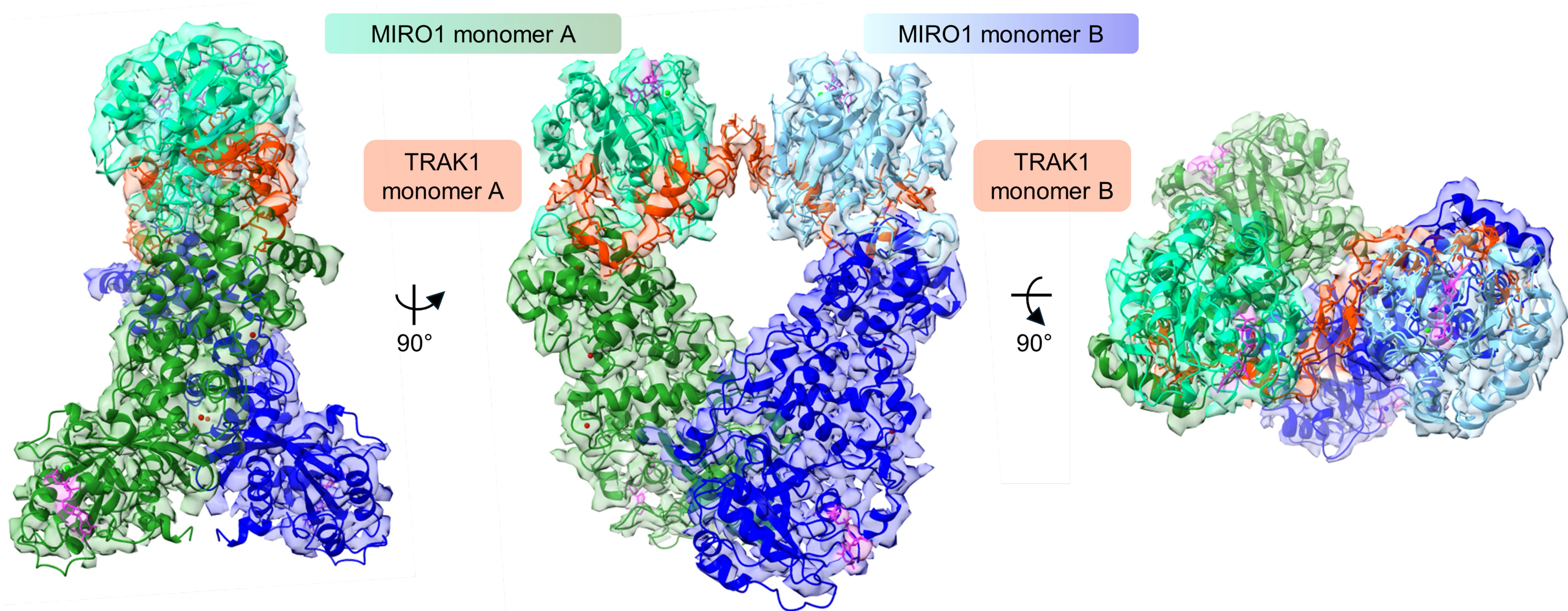
b TRAK1 569-623 -MIRO1 1-591 3.75Å Resolution Map
