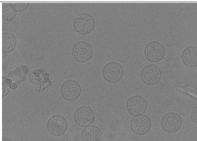
CUS-3 procapsids
